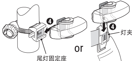
尾灯固定座
