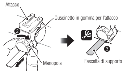
H34 Attacco
