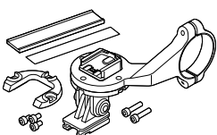
1604110 아웃 프론트 브래킷 2 (OF-200)
